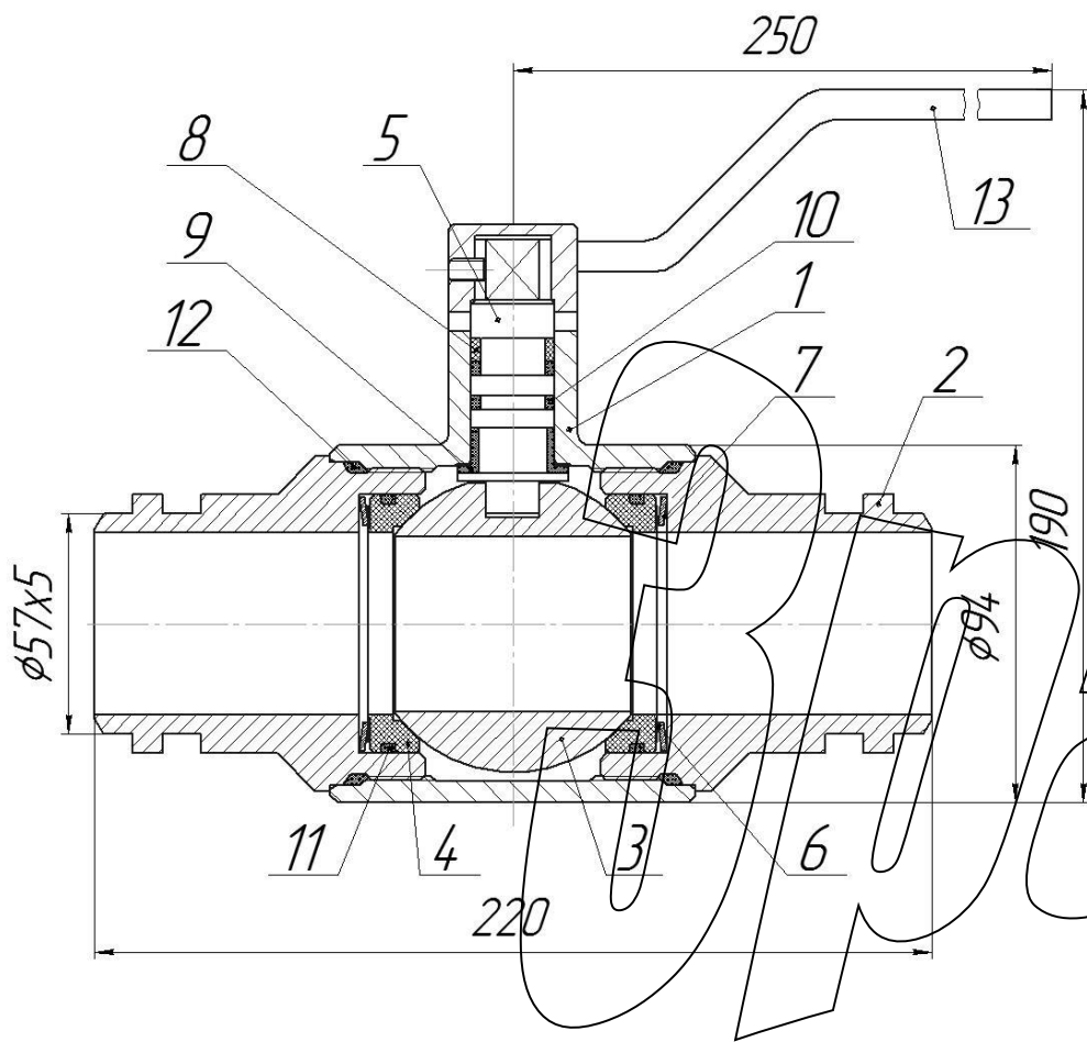
Рисунок 1 – Кран кульовий DN50 PN63 з ручним керуванням (ВКМ.Д-050-063-С-Р-НУ)
